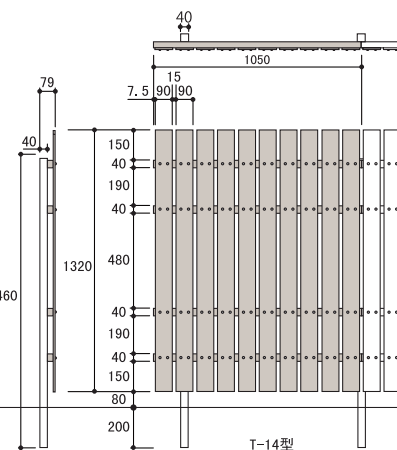
T-14型
