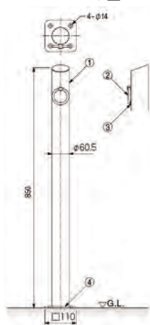
ベースプレート型
