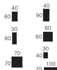
根太・大引・束柱(断面)
