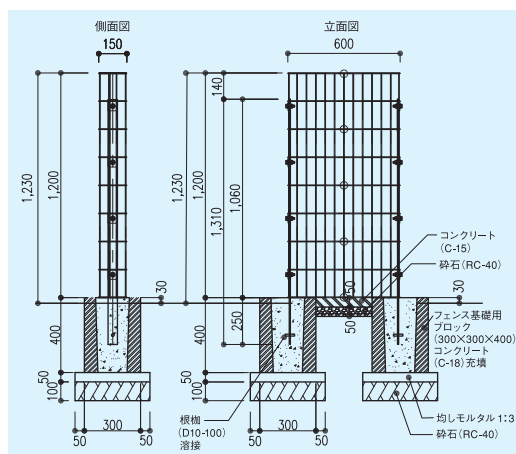
H1200 推奨基礎図
