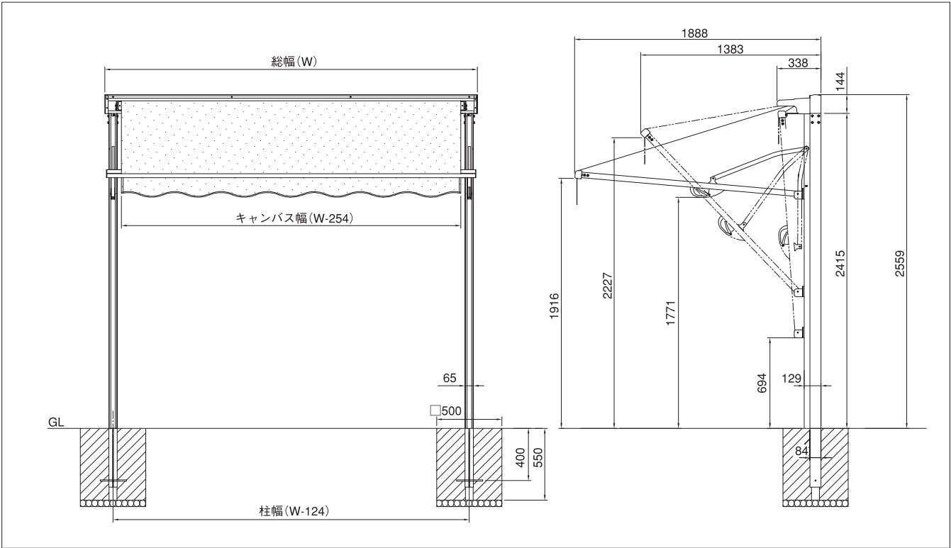
■ 木かげ - 自立型 - 基本寸法図
