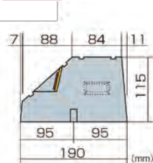
断面図
