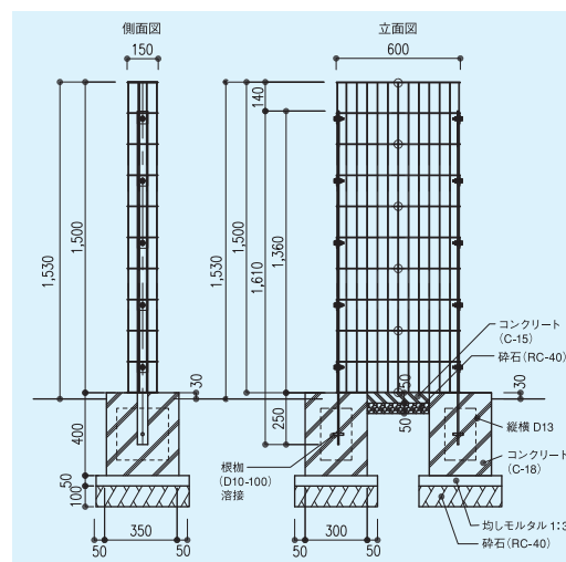
H1500 推奨基礎図
