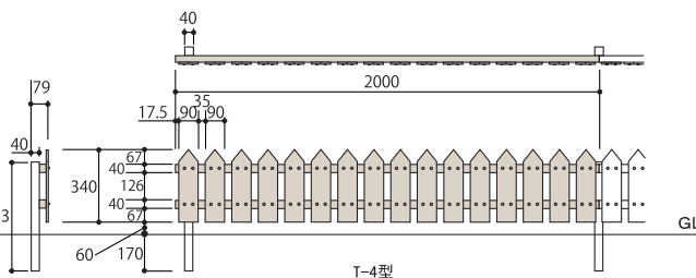
T-4型
